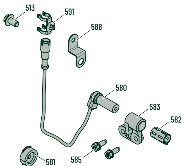
Sensor-Gruppe 05.803.61.73.0 / 74.0
