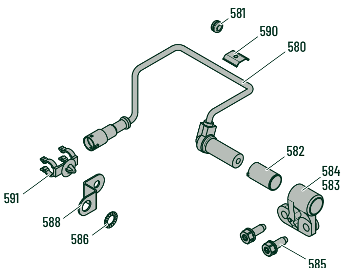
Sensor-Gruppe 05.803.61.73.0 / 74.0
