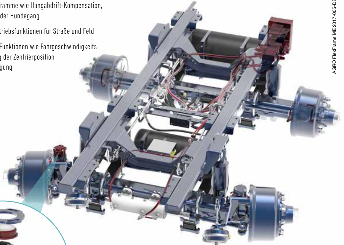
integrierter Sicherheitswinkelgeber in der AGRO Turn Lenkachse
